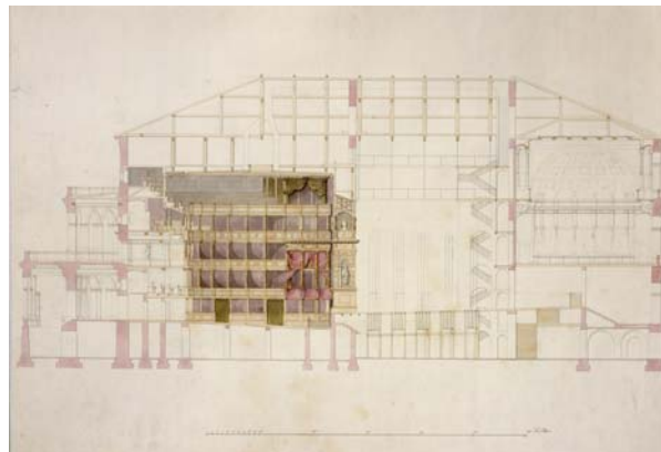
Gottfried Semper (1803 – 1879) Dresden, Erstes Hoftheater Längsschnitt, zweiter Entwurf, um 1838
