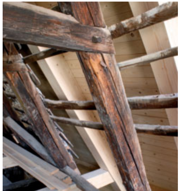
Spätgotischer Dachstuhl mit neuem Überdach, Detail
